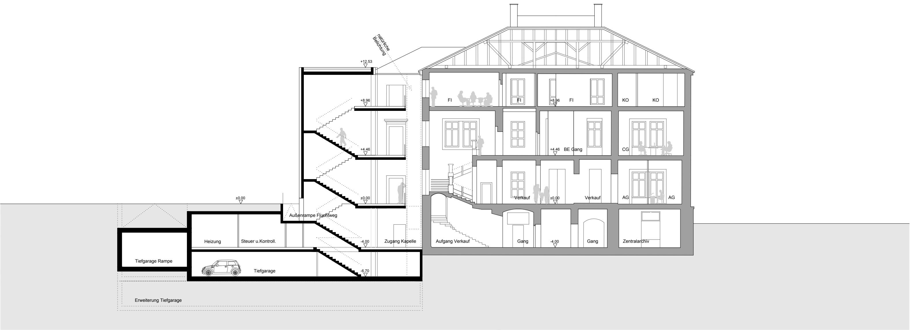
SCHNITT 1-1 1|200
